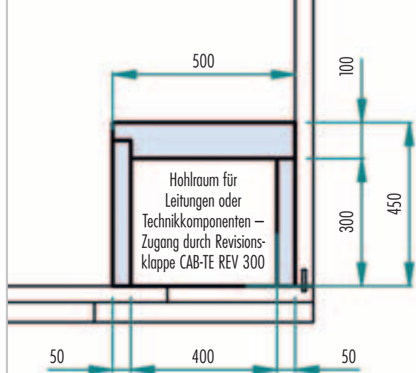
Maße Sitzbank
