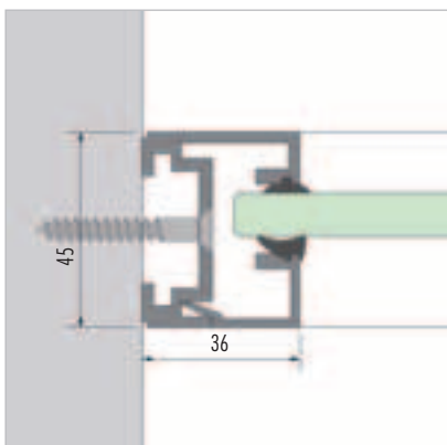
4 Wandprofil, Wandanschluss
