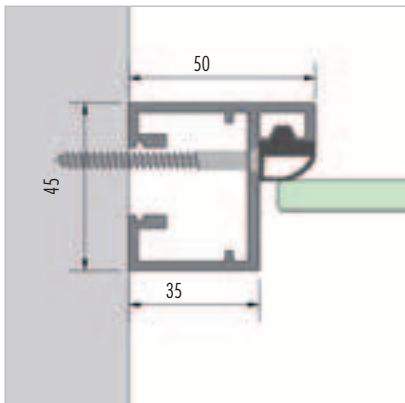
1 Zargenprofil, Wandanschluss
