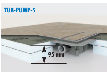
Dimensions sans colle et carrelage
