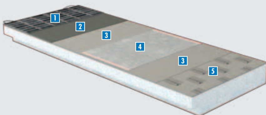
CAB-HE E-BA – bouwschema zitvlakverwarming
